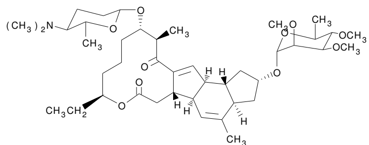
spinosyn D
